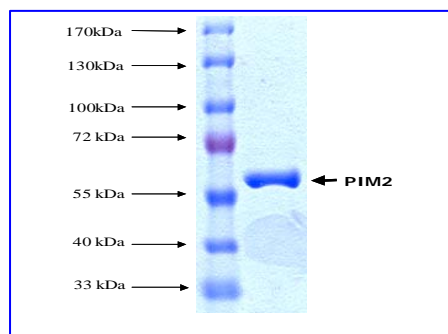
Fig. 2 Pim2 protein gel
